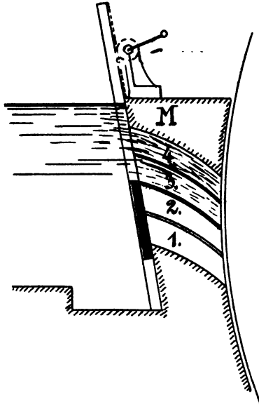
Fig. 18. Kulleneinlauf.
